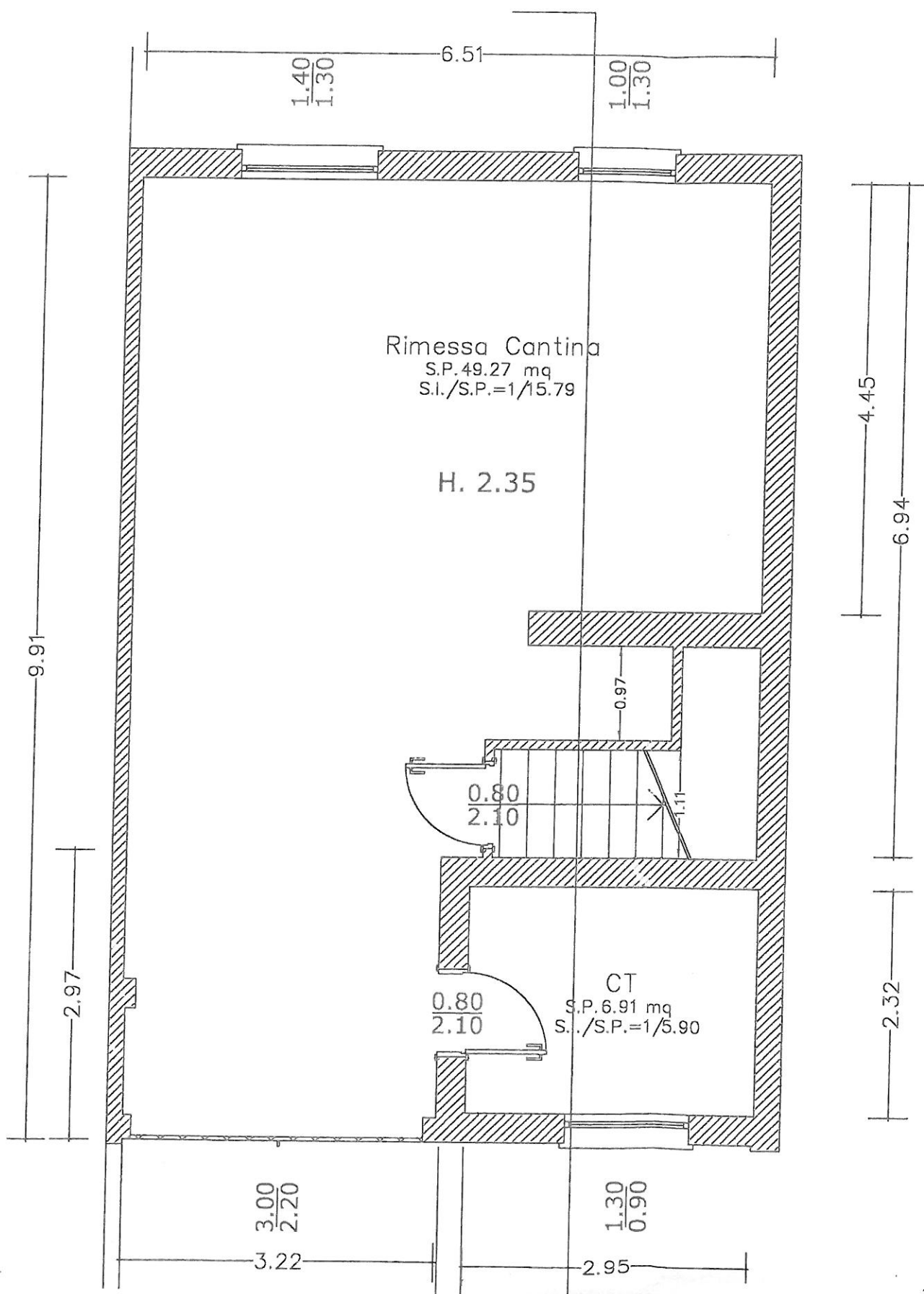
PIANTA PIANO SEMINTERATO
